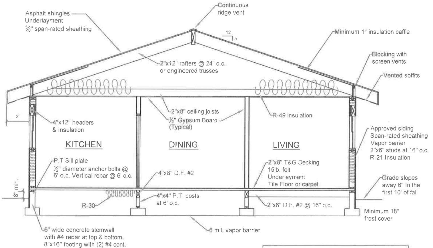
Cross Section SCALE: \frac{1}{4}'' = 1'
